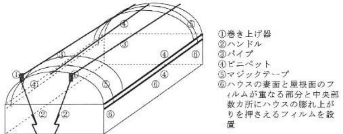
図5 フルオープンハウスの略図（屋根面のフィルムを巻き上げた状態）
