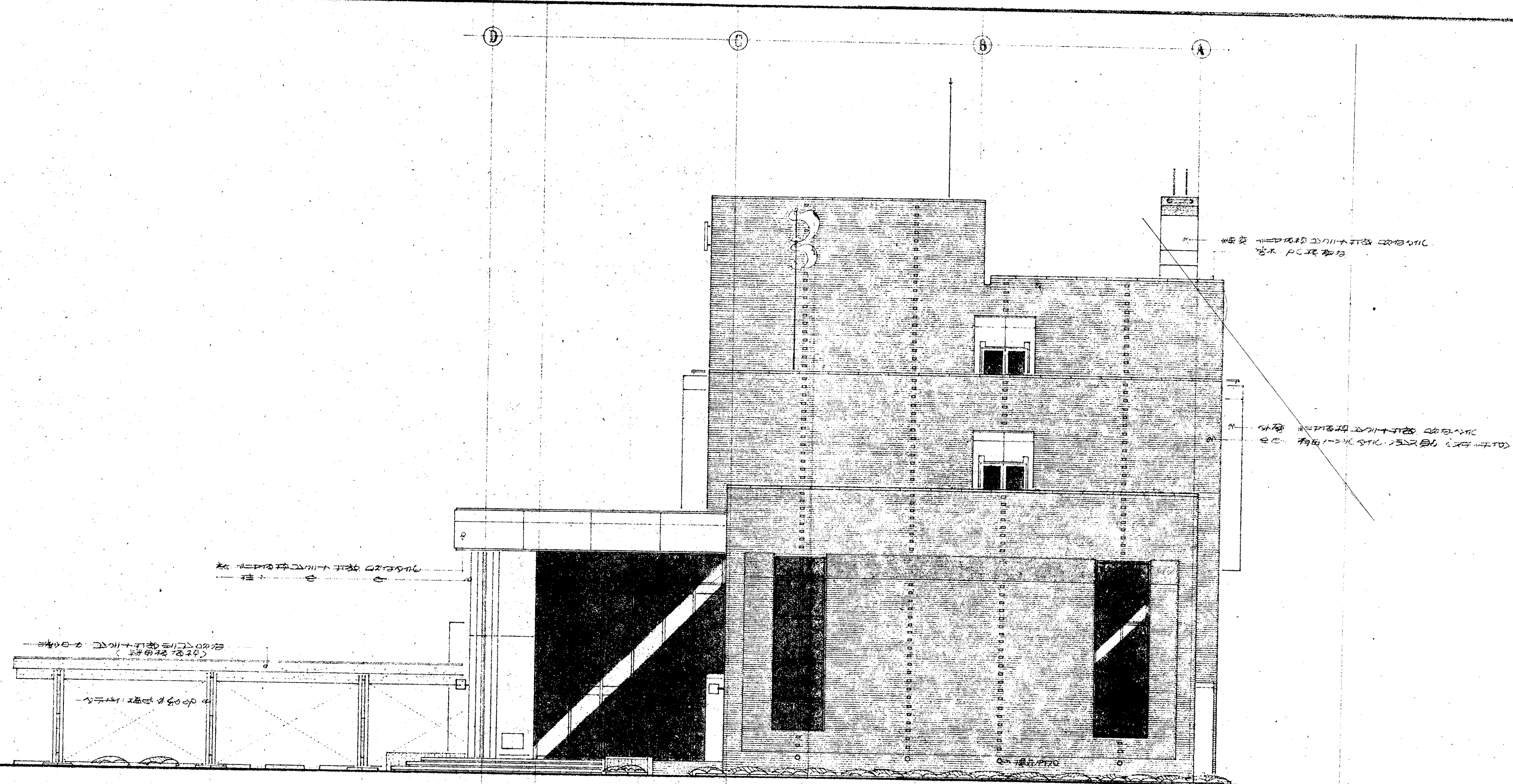
東面立面図 1:100
