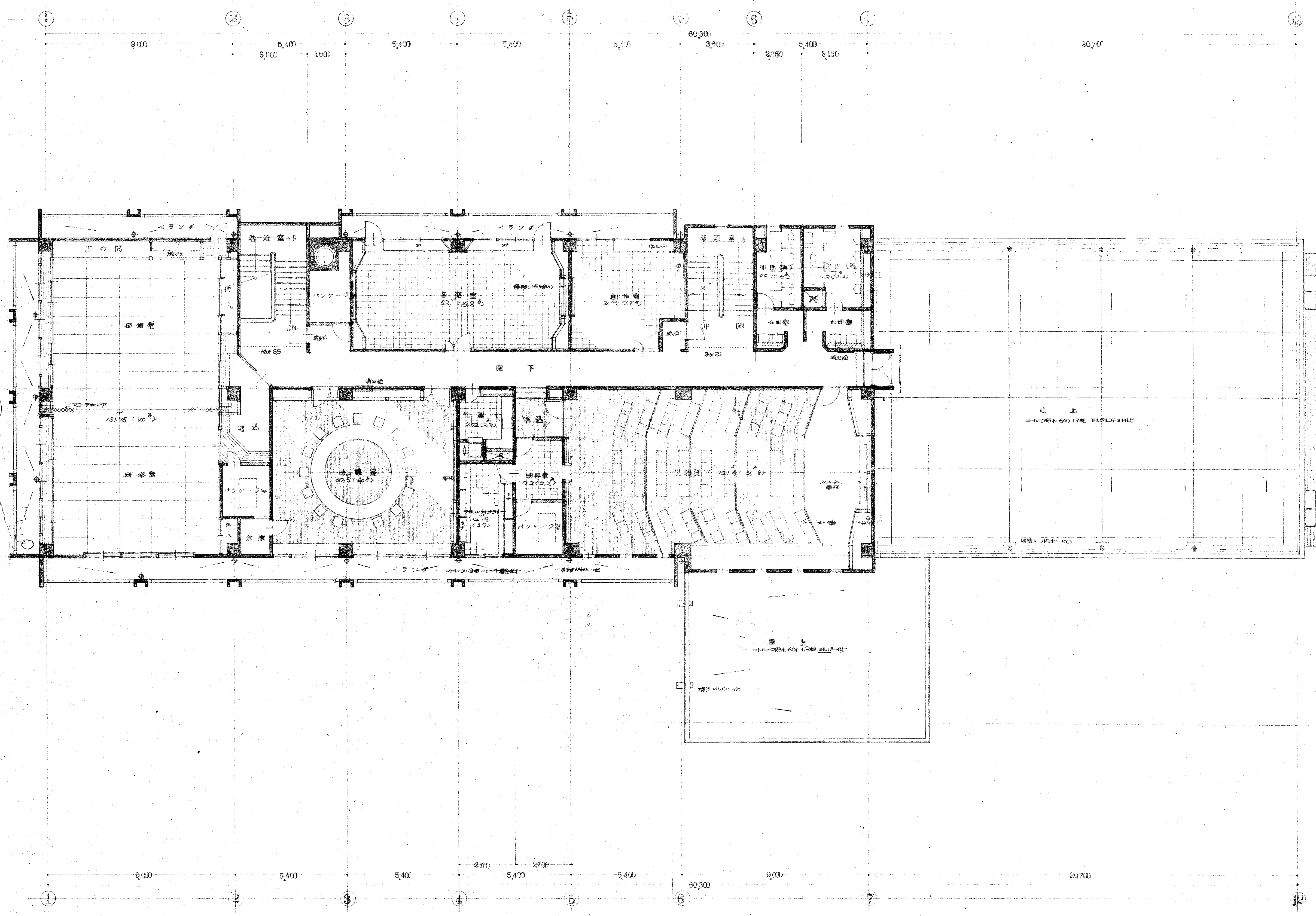
3 階 平 面 図 1/100
