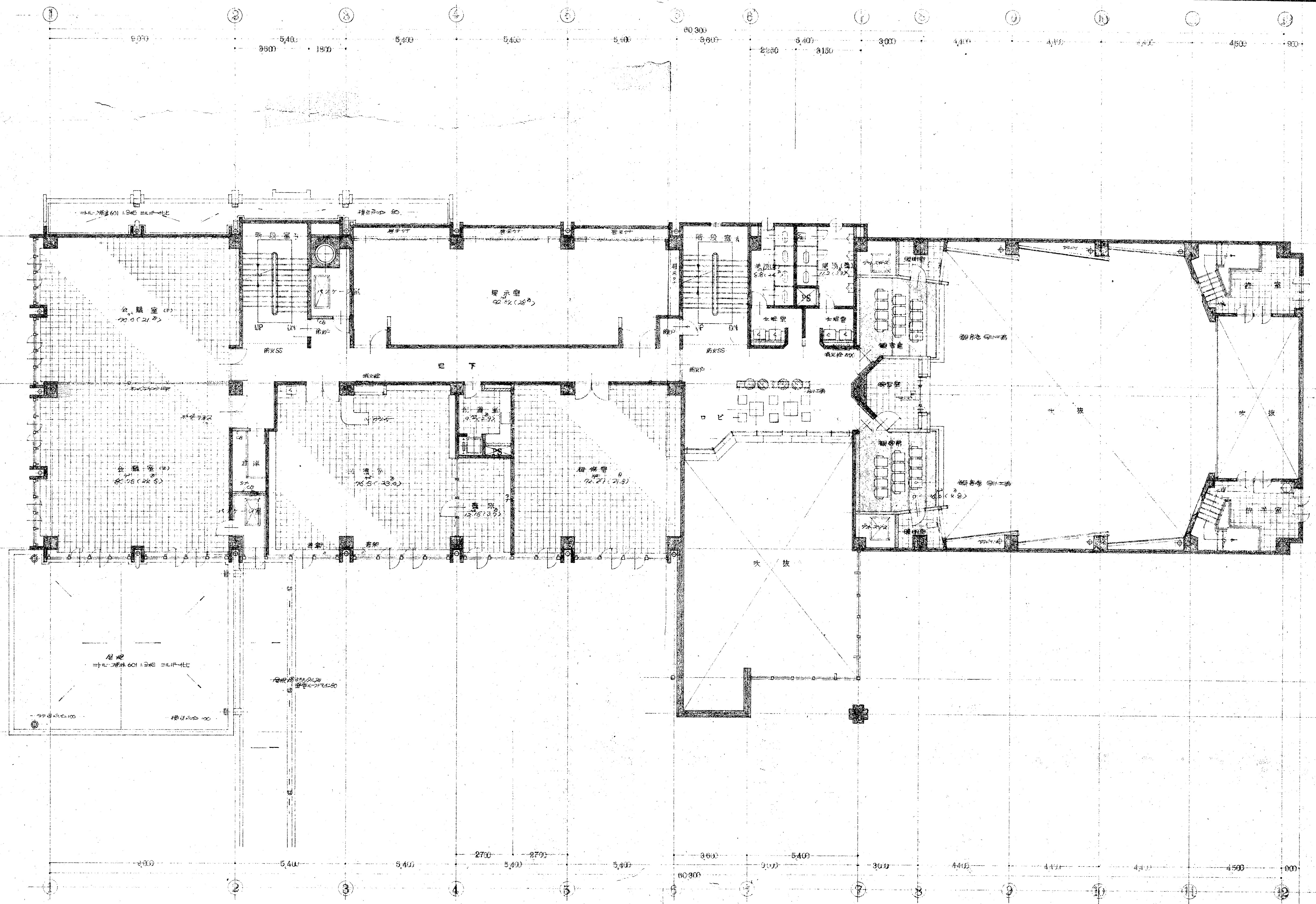
2 樓平面圖 1:100
